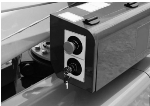
Fig. 64 Nødstopknapp på bælte
