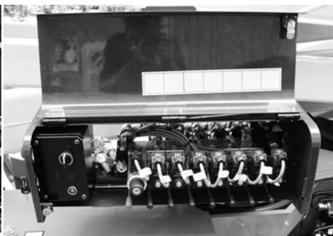
Fig. 61 Hydrauliske jordbetjeninger
