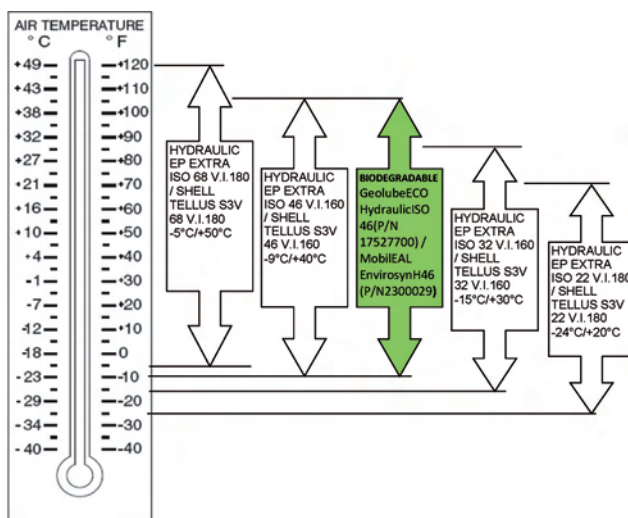
Fig. 152 Olie anvendelsestemperaturer
