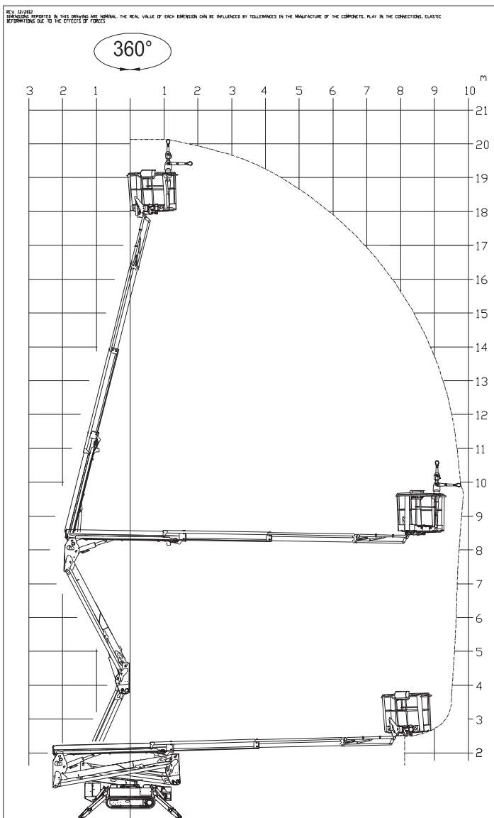
Fig. 83 Arbejdsområde
