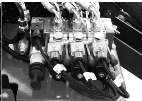
Fig. 80 Styringer på højre fordeler
