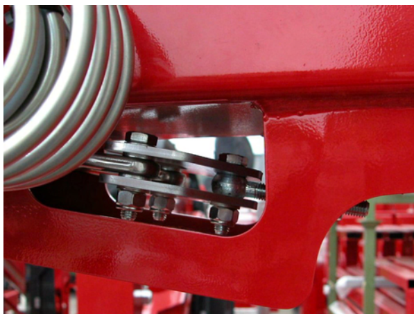
Fig. 174 Vippearm til fastgørelse af returrørene
