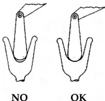
Fig. 173 Eksempel på nedslidte taljer
