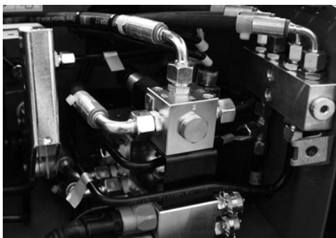
Fig. 142 Luftdelens deviator - bæltedel
